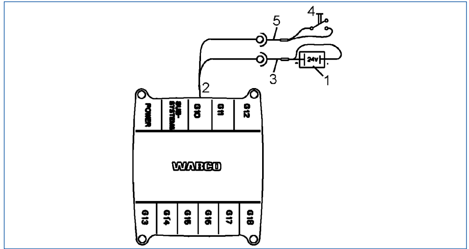
Auszug aus Schema 841 802 250 0 – GIO/ECAS-Funktion mit Batterie
