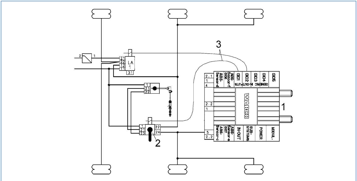
Auszug aus Schema 841 802 150 0
