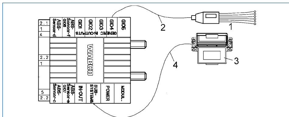
Auszug aus Schema 841 802 157 0
